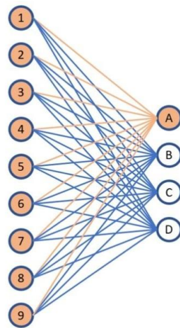
Hình 1.8 Ảnh mô tả cách hoạt động của lớp kết nối đầy đủ
