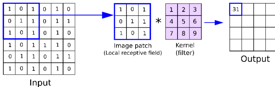
Hình 1.5 Ví dụ về phép tích chập
