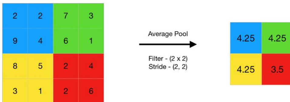
Hình 1.7 Ví dụ về phép gộp trung bình
