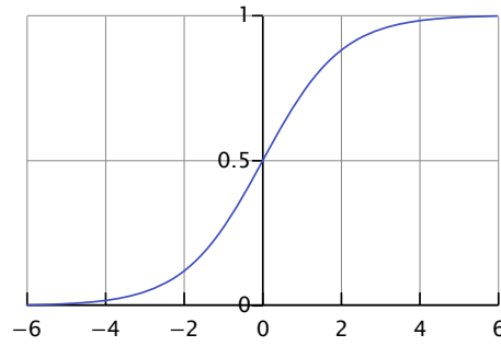
Hình 1.10 Ví dụ đồ thị hàm Sigmoid
