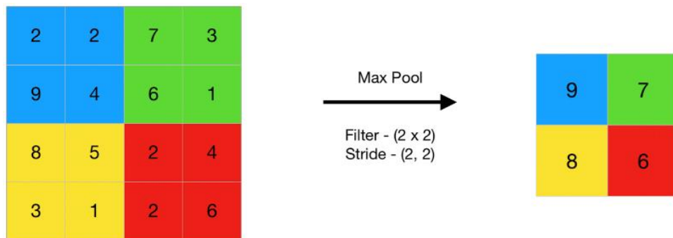
Hình 1.6 Ví dụ về phép toán gộp cực đại
