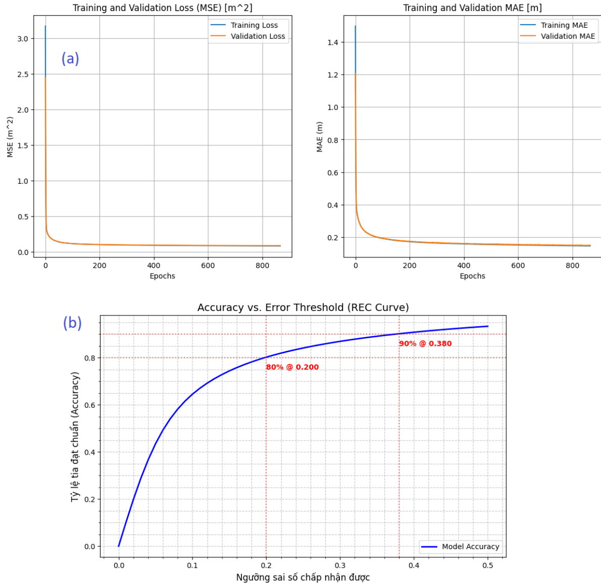
Hình 3.6 Phân tích trực quan hiệu năng mô hình RDC
