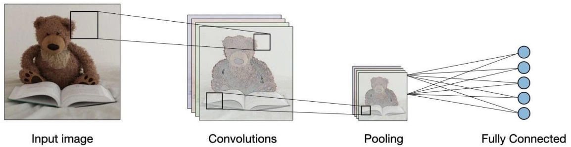
Hình 1.4 Sơ đồ tổng quát mạng nơ-ron tích chập
