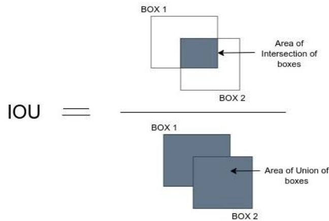
Hình 1.22 Công thức tính IoU
