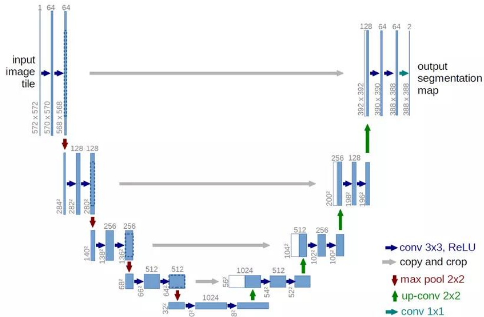
Hình 1.15 Kiến trúc U-Net
