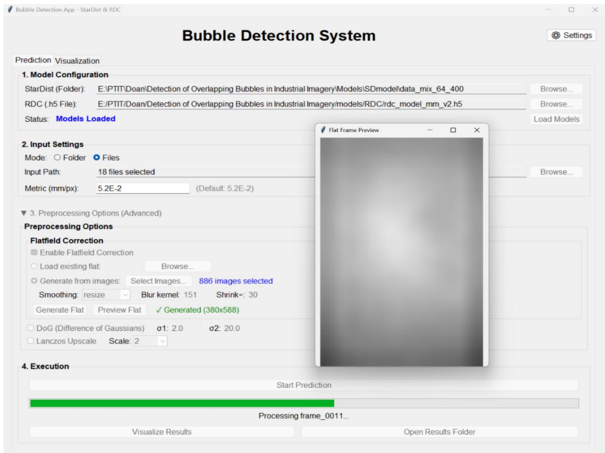
Hình 3.9 Giao diện prediction
