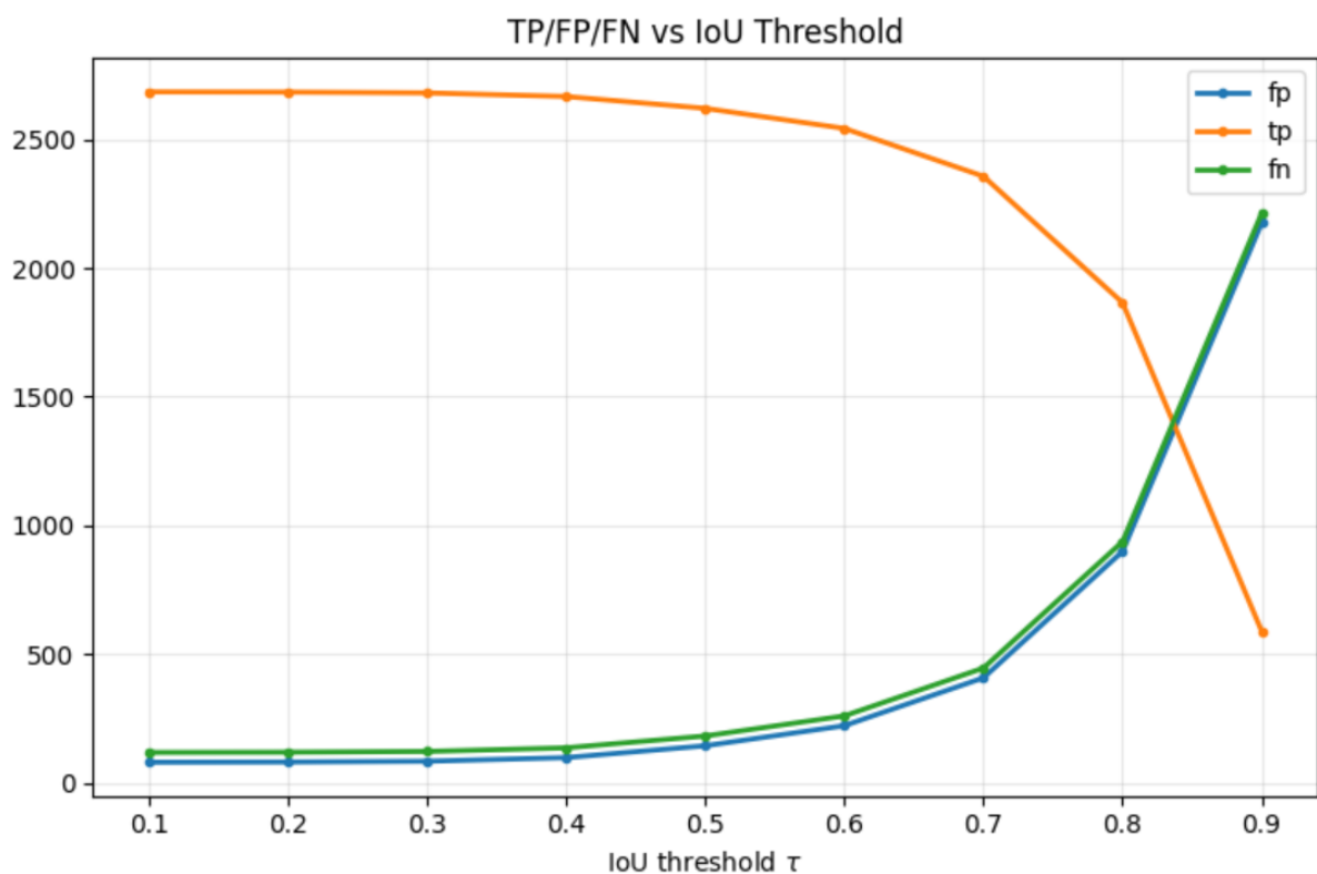
Hình 3.2 Tương quan giữa số lượng TP, FP và FN khi thay đổi ngưỡng đánh giá \tau
