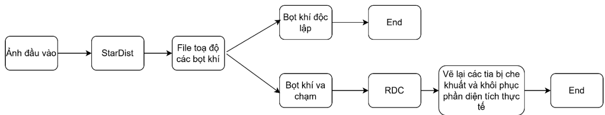
Hình 1.20 Mô tả phương pháp áp dụng StarDist + RDC
